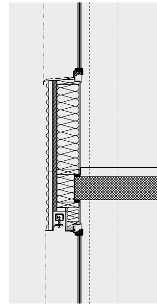
Beton/HSB_Stütze vor Aussenwand
