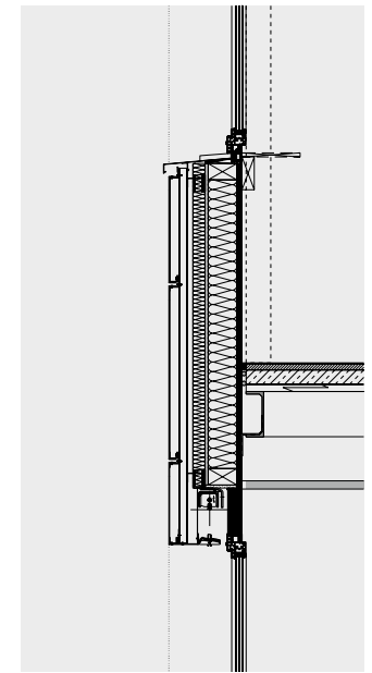
Stahl/HSB_ohne Installationsebene
